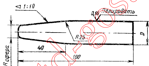
Черт. 31
