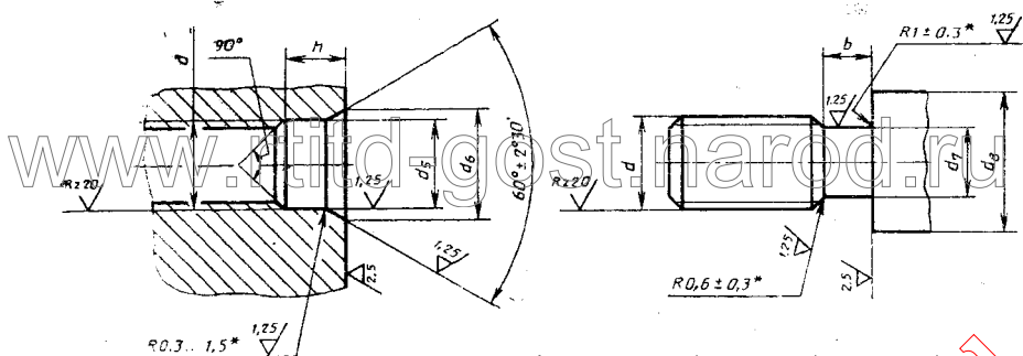
Черт. 24
