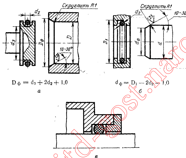
Черт. 25
