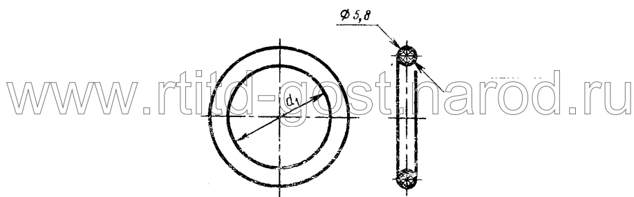
Черт. 8
