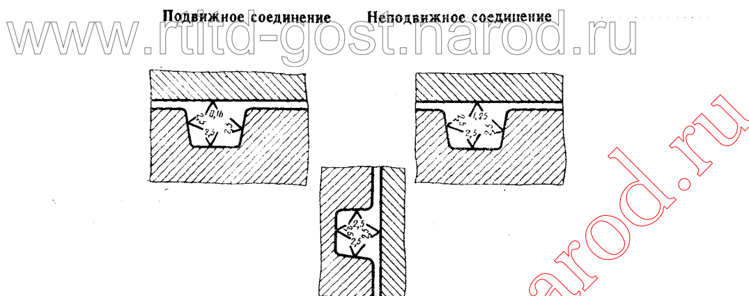
Торцовое соединение
