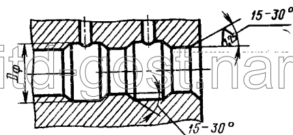
Черт. 26
