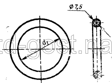
Черт. 9
