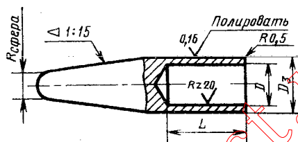
Черт. 27
